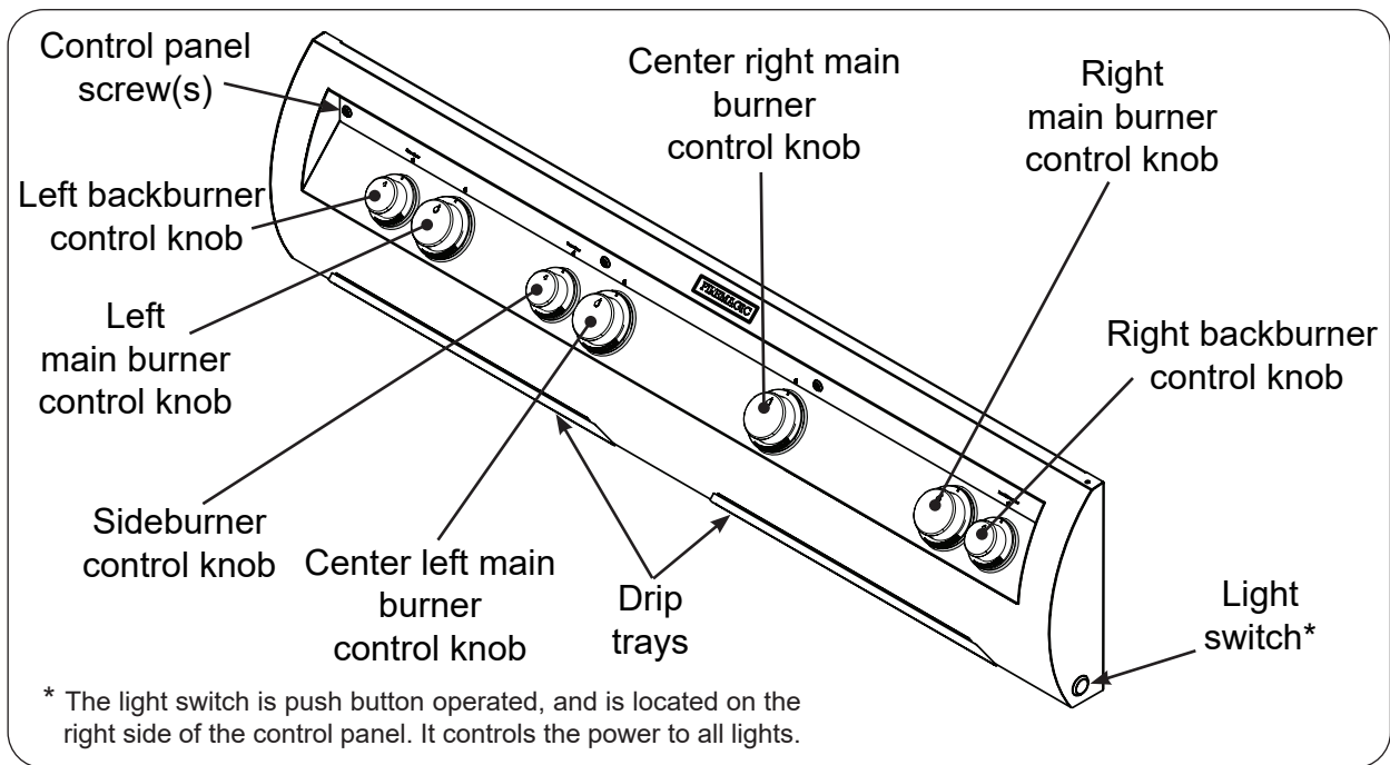
Fig. 25-1 E1060s controls
