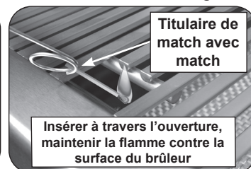
Fig. 28-3 Eclairage manuel via porte allumette
