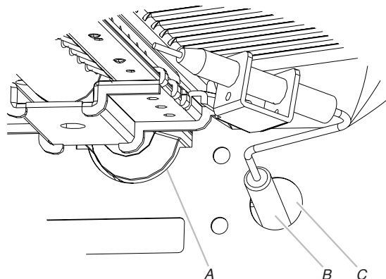
A. Trous de l'injecteur du brûleur de cuisson au gril B. Électrode du brûleur de cuisson au gril C. Trous de l'électrode du brûleur de cuisson au gril
