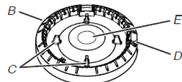
A. Chapeau de brûleur B. Base du brûleur C. Tiges d'alignement D. Électrode d'allumage E. Ouverture du tube d'arrivée de gaz
