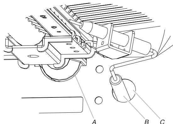
A. Trous de l'injecteur du brûleur de cuisson au gril B. Électrode du brûleur de cuisson au gril C. Trous de l'électrode du brûleur de cuisson au gril
