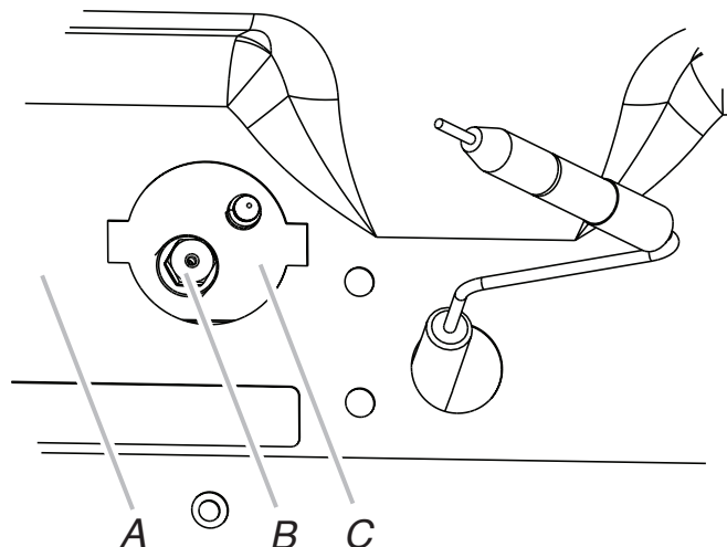
A. Arrière du four B. Injecteur du brûleur de cuisson au gril C. Trous de l'injecteur du brûleur de cuisson au gril
