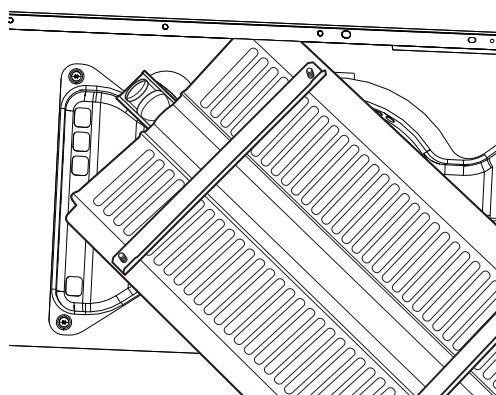
Le brûleur de gril pend à l'arrière du four
