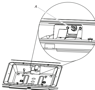
A. Gicleur de gaz propane
