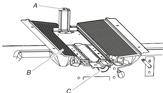
A. Vis du brûleur de cuisson au gril B. Brûleur du gril C. Trous de l'injecteur du brûleur de cuisson au gril
