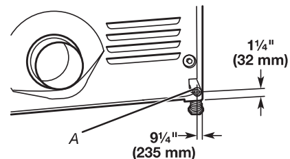
A. Conduit NPT de la sécheuse de 3/8"
