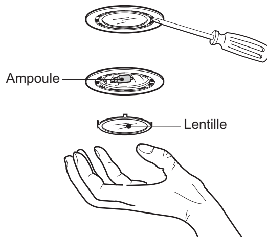
Figure 28 : Remplacement des ampoules halogènes
