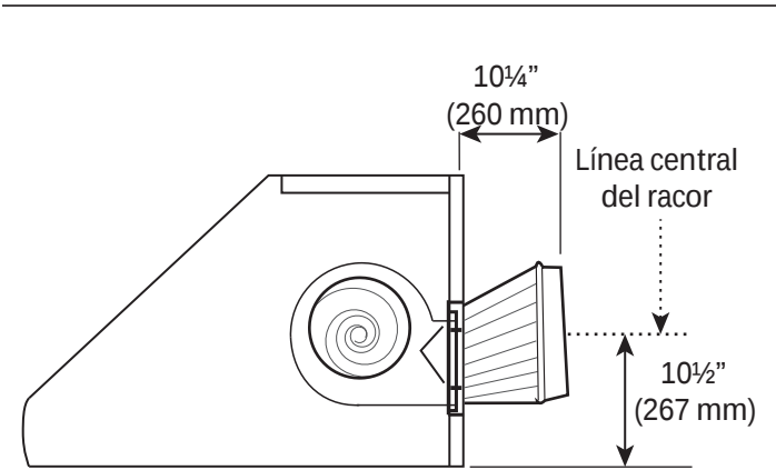
Figura 10: Línea central del racor para una salida horizontal
