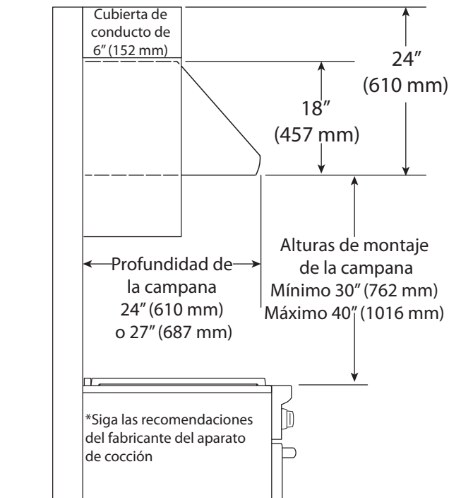
Figura 6: Instalación típica de la campana
