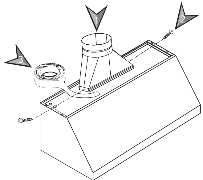
Figura 5: Conexión del racor
