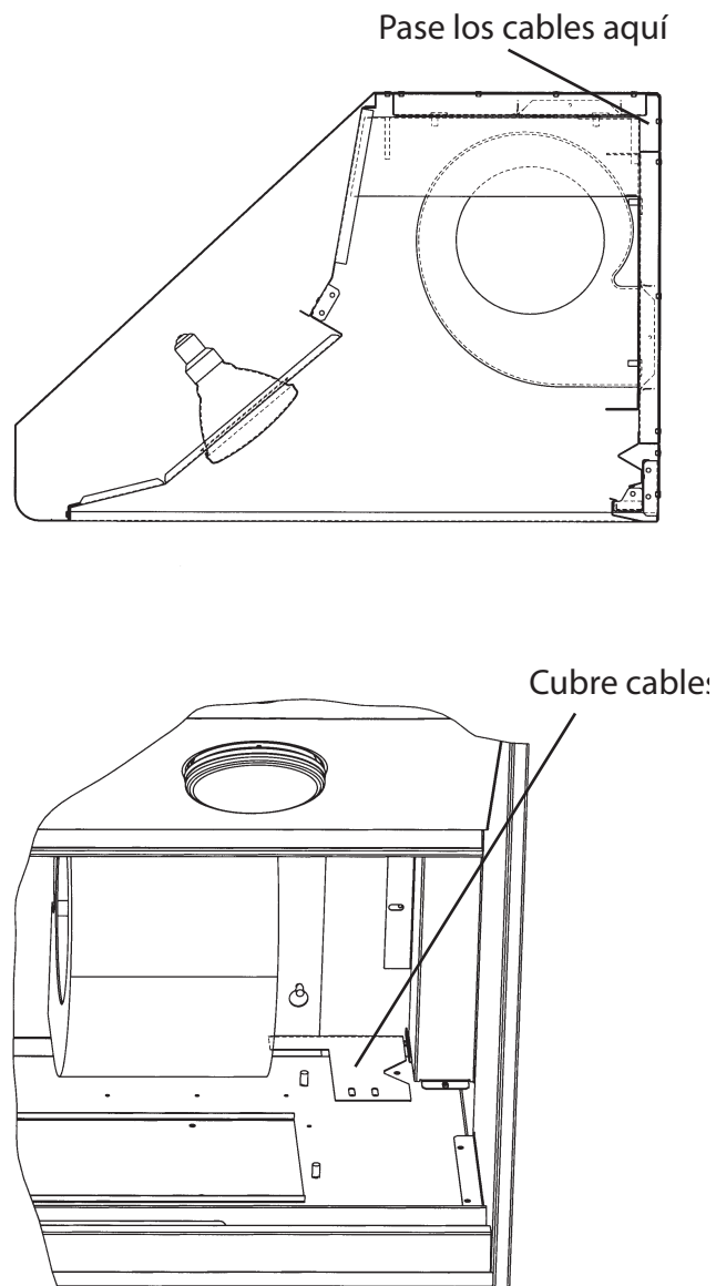
Figura 25: Salida horizontal
