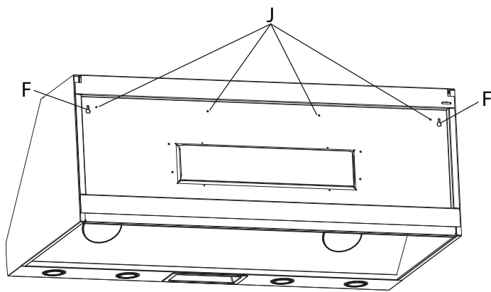
Figura 13: Ubicación de las muescas en forma de ojo de cerradura
