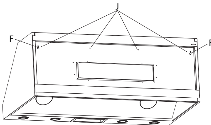
Figure 13 : Emplacements des encoches en trou de serrure
