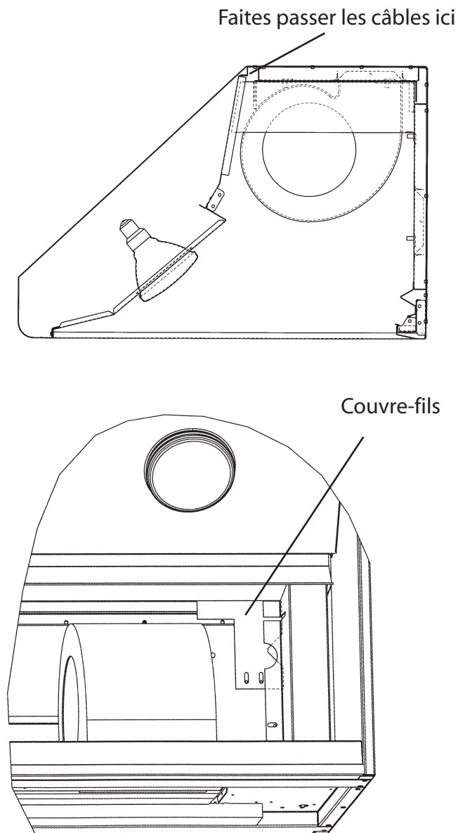
Figure 24 : Débouché vertical
