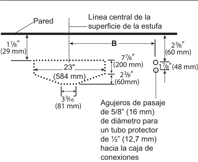
Figura 16: Ubicación del racor y del tubo protector
