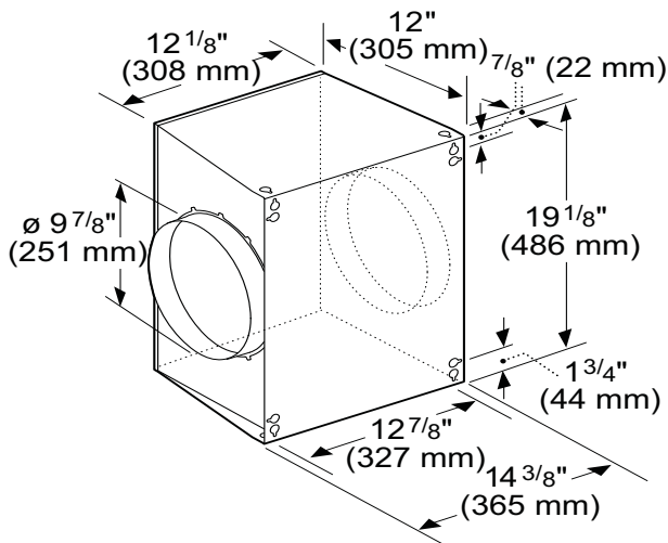
Figura 22: Ventilador en línea VT1010D
