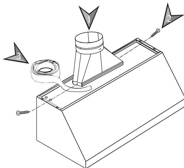
Figure 5 : Connexion du raccord
