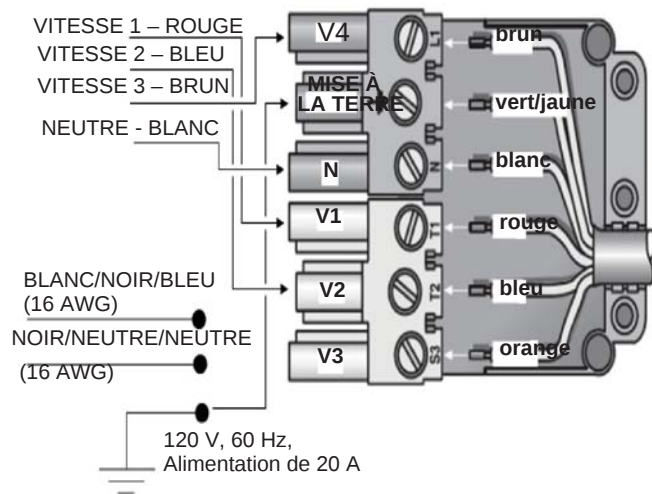
Figure 21 : Câblage de la hotte avec un ventilateur à distance
