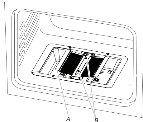
A. Oven baffle B. Oven baffle nuts
