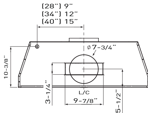
Vue arrière
