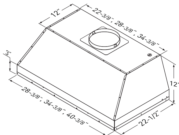
Vue 3/4
