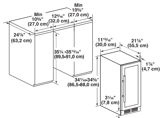
Dimensions critiques pour modèles de 15"
