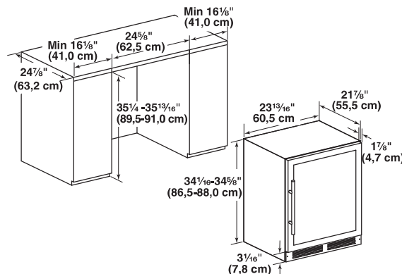
Dimensions critiques pour modèles de 24"
