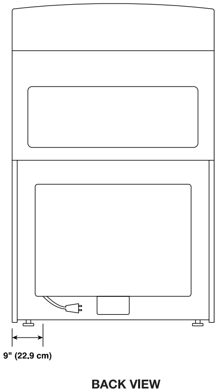
WIDTH TO ELECTRICAL CONDUIT
