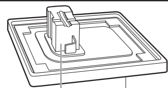
Soporte de base de espuma Base de cartón
