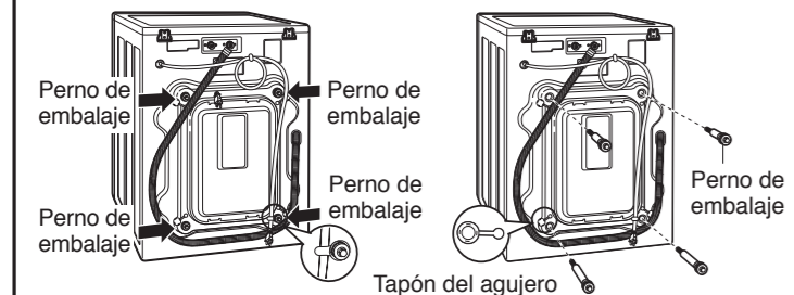
Perno de embalaje Tapón del agujero
