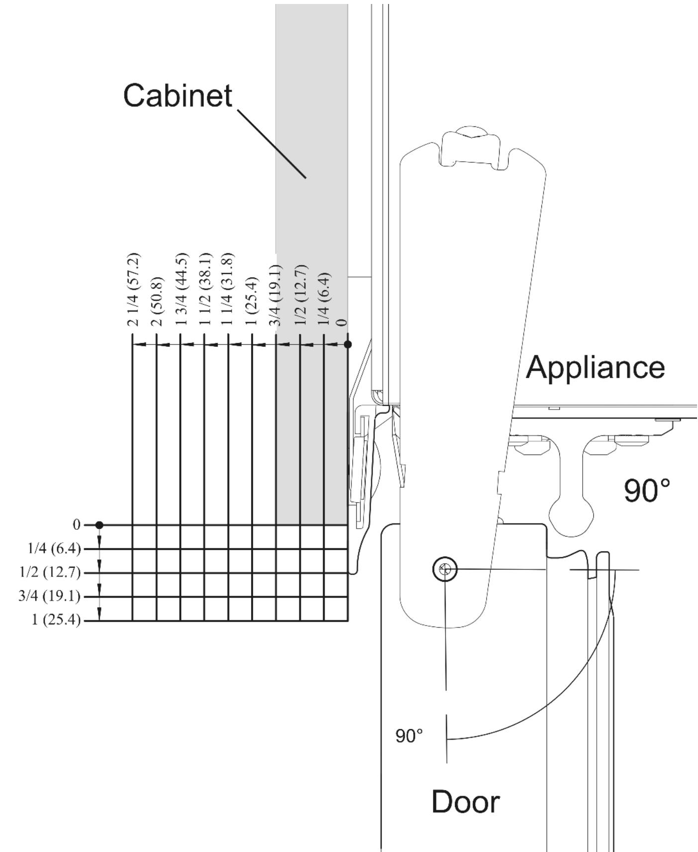
Fig. 10 90°, hinges on left
