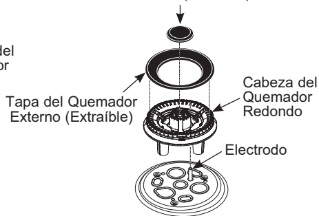
Quemador de múltiples anillos (en algunos modelos)
