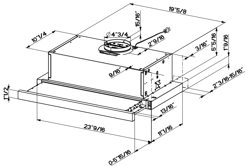
CAMPANA EXTRACTORA DE 24"
