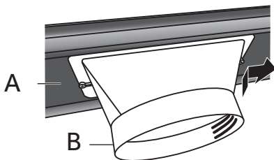
(A) Panel principal de la ventana (B) Boquilla de escape (1 o 2 dependiendo del modelo)
