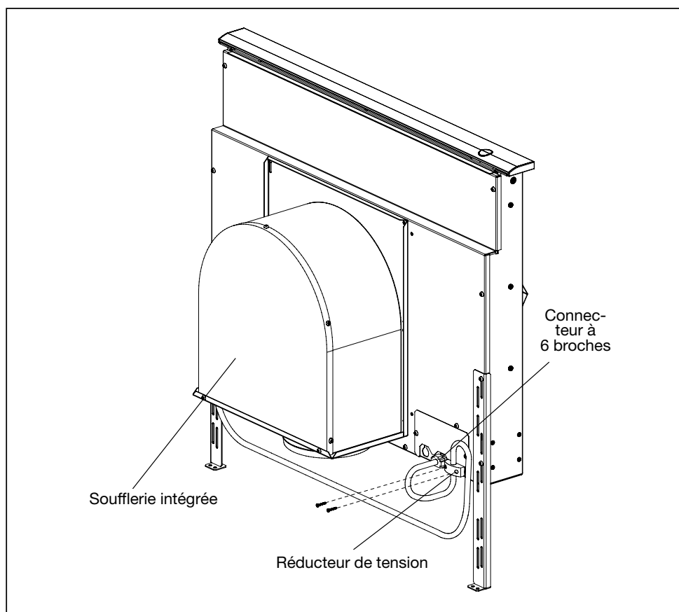
Fig. 9 – Soufflerie intégrée
