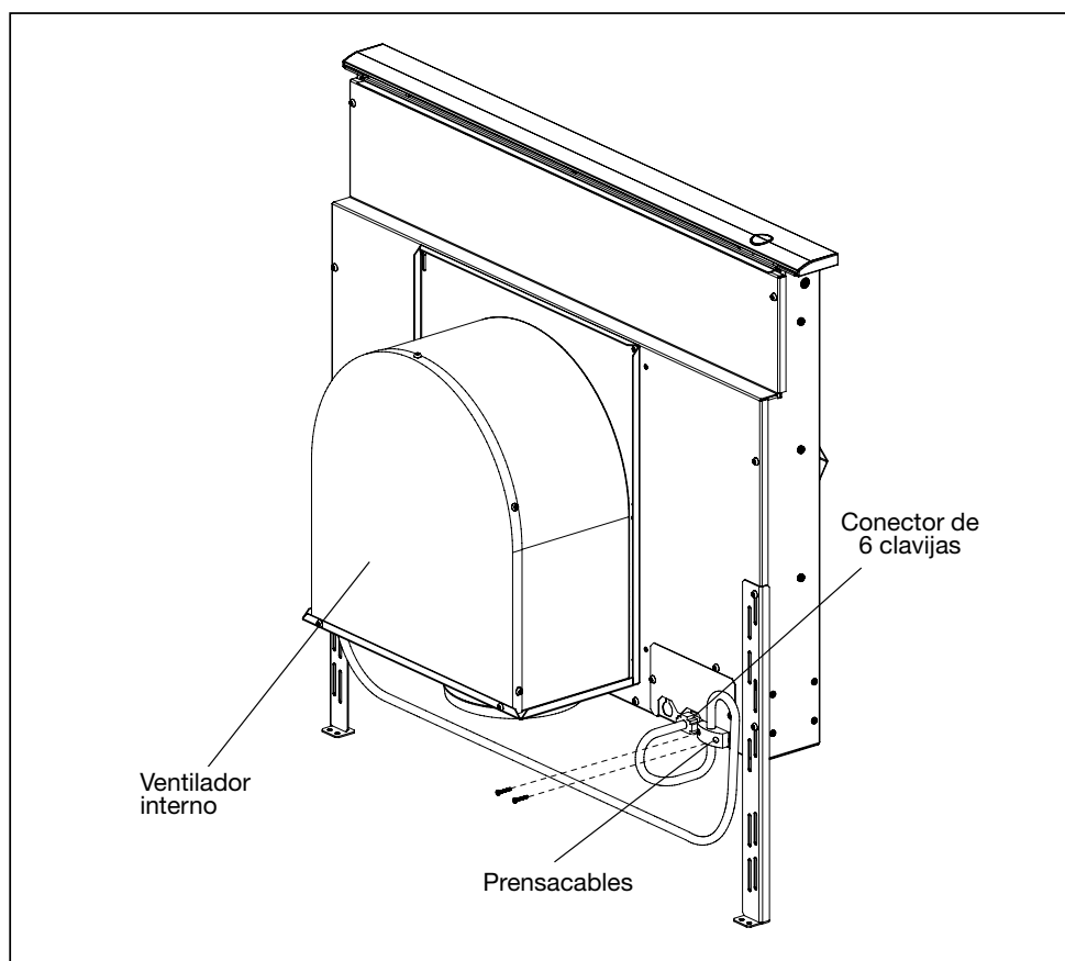
Fig. 9 – Ventilador interno
