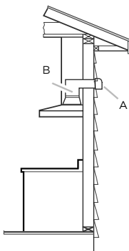
Ventilación a través de pared
