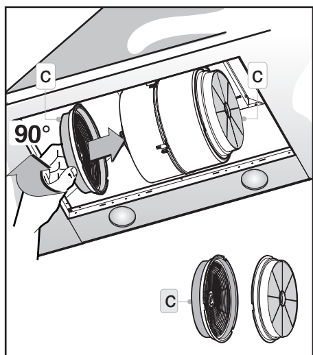
Fig.9: Los filtros C deben aplicarse a la unidad aspirante que se encuentra dentro de la campana, centrándolos en la misma y girándolos 90° hasta oír el clic de bloqueo.
