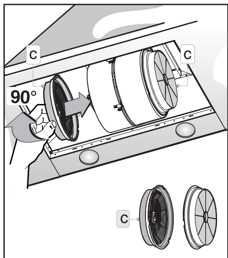
Fig.9: Les filtres C doivent être appliqués au groupe aspirant situé à l'intérieur de la hotte en les plaçant au centre de celui-ci et en les tournant de 90 degrés jusqu'au déclic de blocage.
