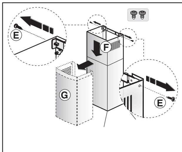
Fig.1: Quitar los 2 tornillos E y hacer bajar la chimenea superior F en el interior de la chimenea inferior G . Quitar las dos chimeneas F-G apoyándolas cuidadosamente en una superficie.
