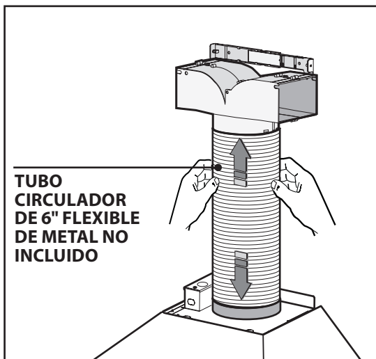
Fig.6: Una vez que se introduzca el deflector en la brida y se fije a la pared, conecte el tubo flexible ( TUBO CIRCULADOR DE 6" FLEXIBLE DE METAL NO INCLUIDO ) al deflector, utilice una cinta para sellar.
