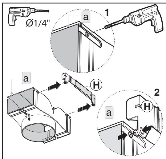
Fig.4: Prendre le déviateur d'air A et faire deux trous comme indiqué sur la figure (diamètre trou: 1/4" pouces). Après avoir effectué les deux trous, fixer le déviateur d'air A à l'étrier de fixation des cheminées H .
