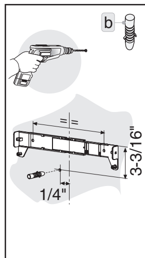
Fig.2: Marcar y efectuar un agujero de fijación a 1/4" pulgadas del centro de la brida e introducir el taco de expansión.
