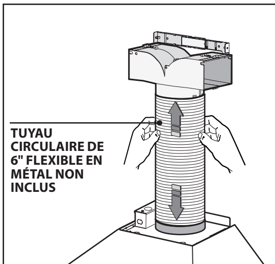
Fig.6: Après avoir introduit le déflecteur dans l'étrier et l'avoir fixé au mur, raccorder le tuyau flexible ( TUYAU CIRCULAIRE DE 6" FLEXIBLE EN MÉTAL NON INCLUS ) au déflecteur, utiliser du ruban isolant pour sceller.
