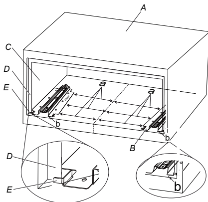
A. Gabinete B. Rieles C. Pared lateral D. Taco lateral E. Tapón
