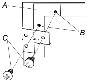
A. Taco B. Orificio piloto C. Tornillo de cabeza redonda para madera n.º 7-16 x 7/16"
