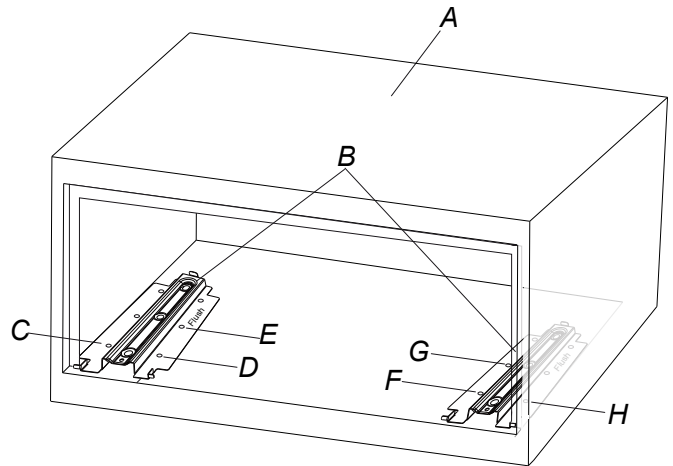
A. Gabinete B. Rieles C. Orificio C en el riel izquierdo D. Orificio D en el riel izquierdo E. Orificio E en el riel izquierdo F. Orificio F en el riel derecho G. Orificio G en el riel derecho H. Orificio H en el riel derecho
