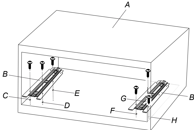
A. Gabinete B. Rieles C. Orificio C D. Orificio D E. Orificio E F. Orificio F G. Orificio G H. Orificio H
