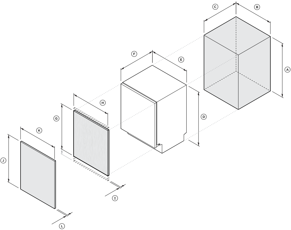
VUE ISOMÉTRIQUE ÉCLATÉE
