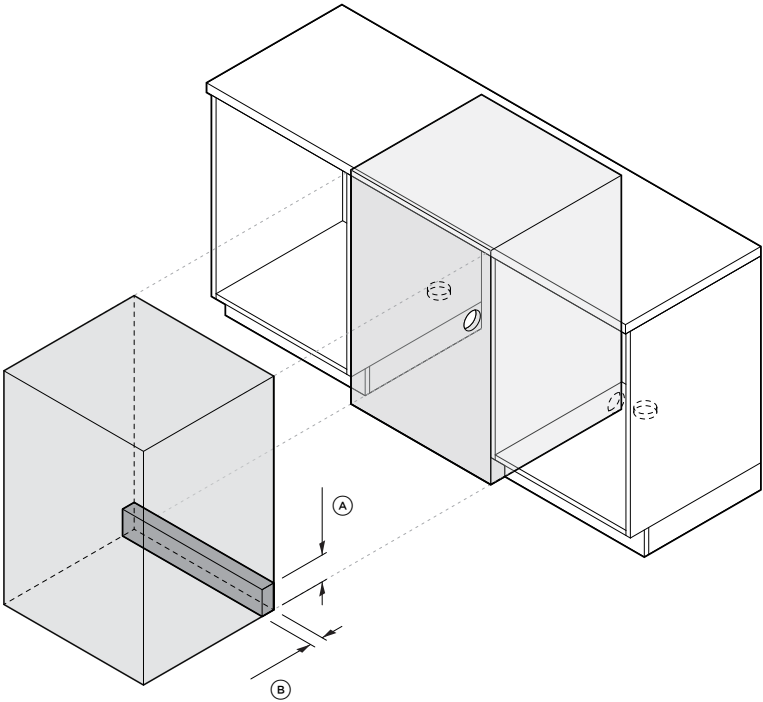
VUE ISOMÉTRIQUE ÉCLATÉE CAVITÉ ET ARMOIRES
