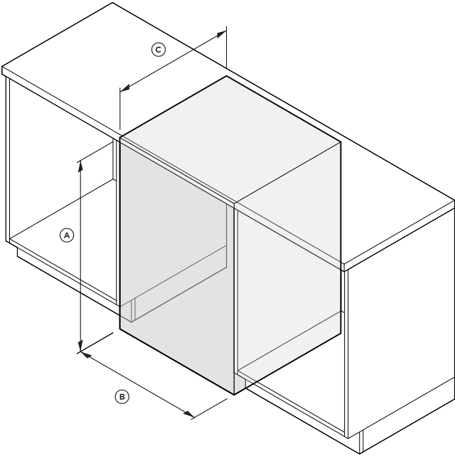
VUE ISOMÉTRIQUE
