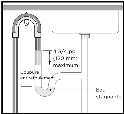
VUE DÉTAILLÉE INSTALLATION DE LA CONDUITE VERTICALE
