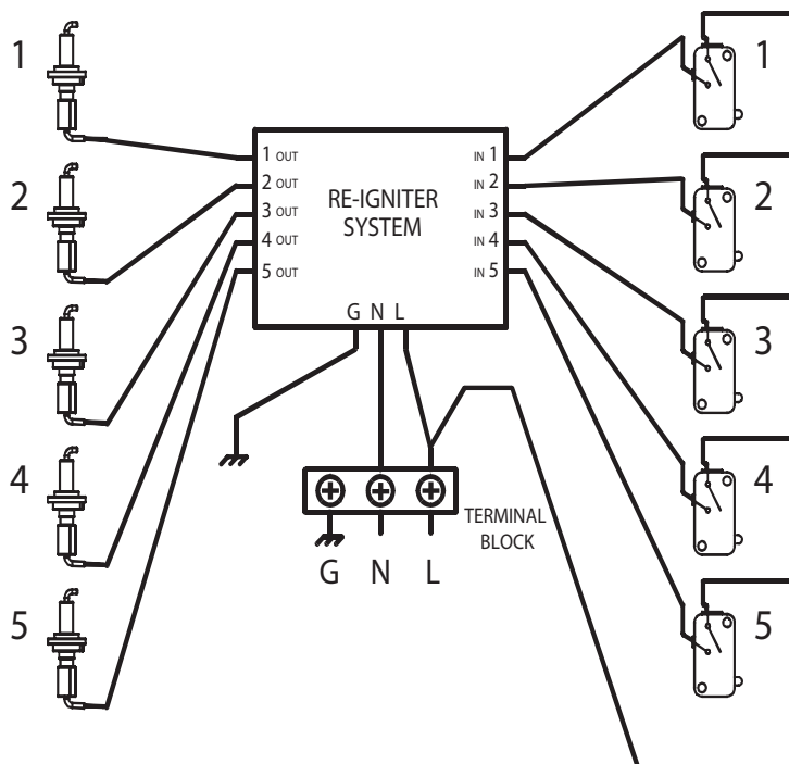
Figure 16. Schéma électrique (5 zones)
