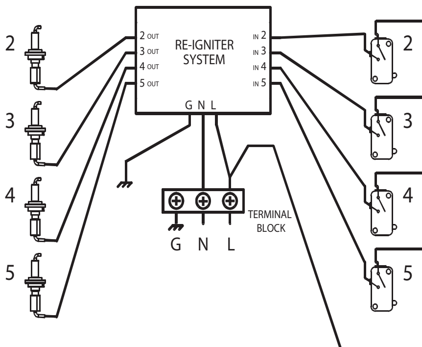
Figure 15. Schéma électrique (4 zones)
