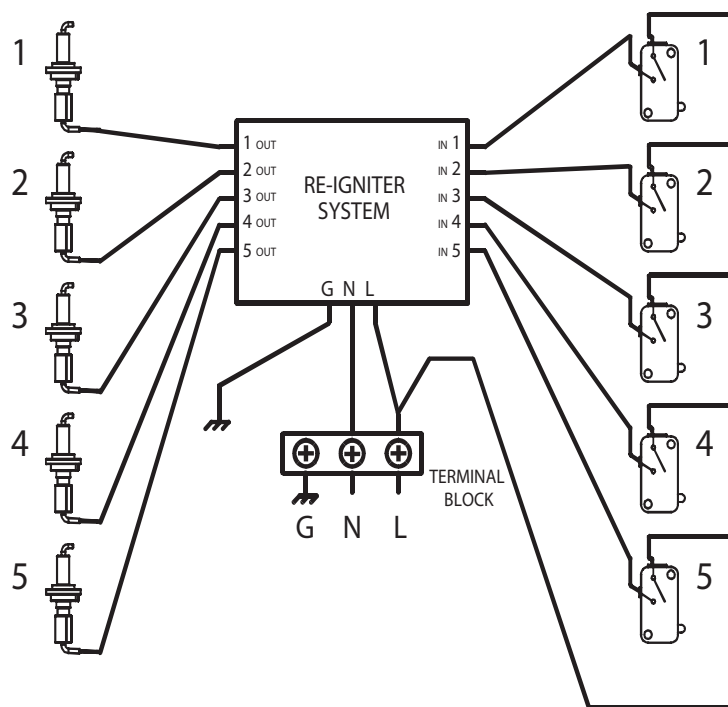
Figura 16. Diagrama eléctrico (5 zonas)
