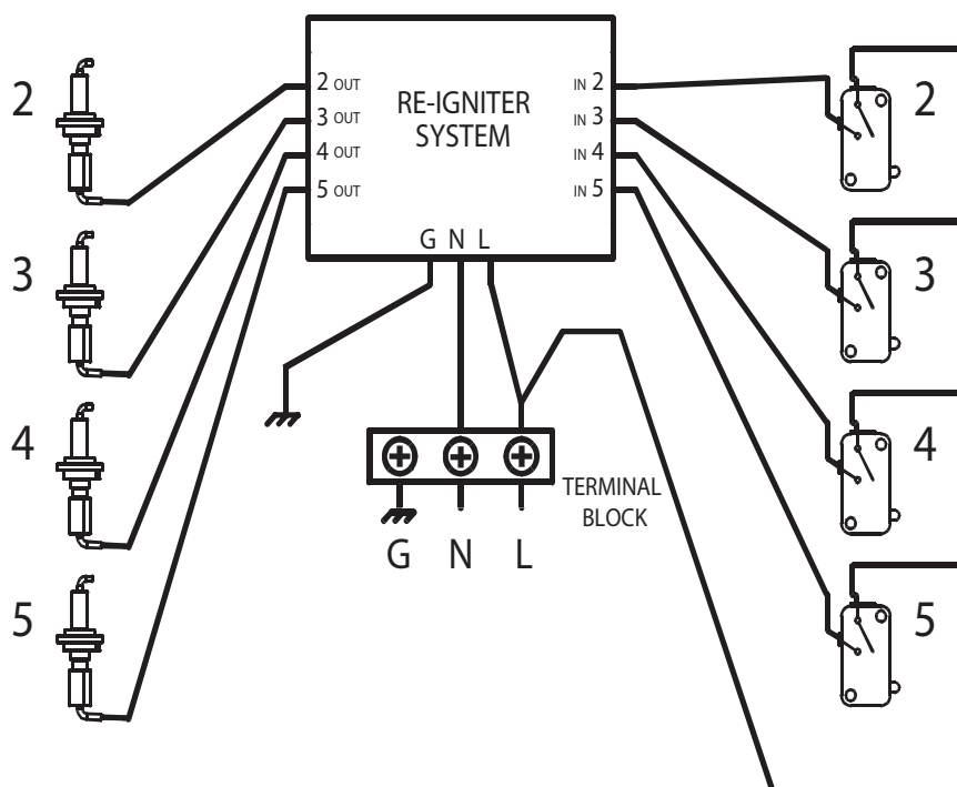
Figura 15. Diagrama eléctrico (4 zonas)
