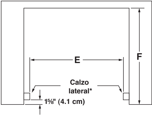
VISTA SUPERIOR
