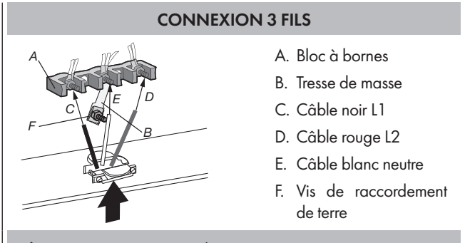
3-CÂBLAGE DU CIRCUIT DE DÉRIVATION (US seulement)
