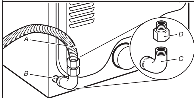
A. Raccord flexible de gaz de 3/8" C. Coude de 3/8" par 3/8" B. Conduit de la sècheuse de 3/8" D. Adaptateur entre le conduit et le joint conique de 3/8"
