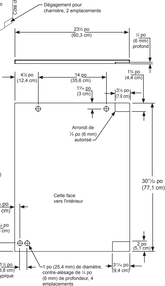
Figure 15 Porte à charnières à gauche Appareil de largeur 24 po (61 cm)
