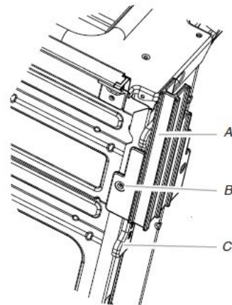
A. Pied avant B. Vis n° 8-18 x 3/8" C. Cale d'espacement
