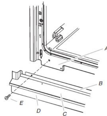
A. Châssis du four B. Support de l'évent C. Évén du four D. Garniture de l'évent inférieur E. Vis n° 8-18 x \frac{3}{8} po (9,5 mm)
