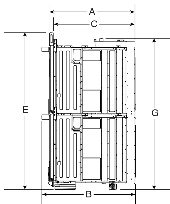
VUE LATÉRALE
