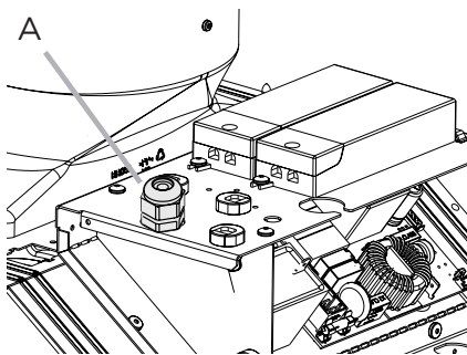
A. \frac{1}{2} " Conduit connector
