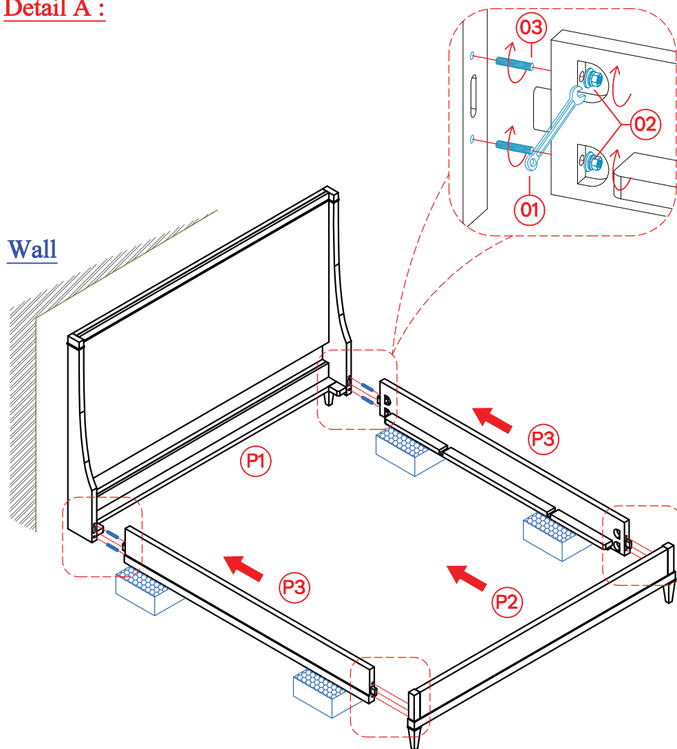
Detail A :
