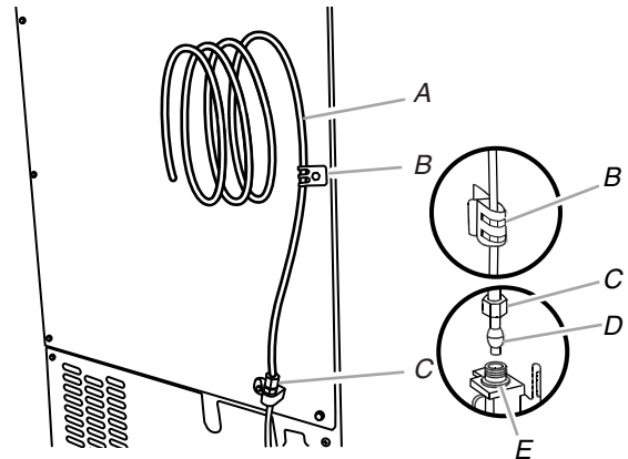
A. Tubería de cobre de 1/4"
