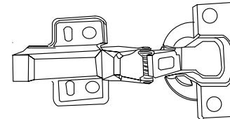
* x4 RP301603-HINGE1 Center Door Hinge Charnière de porte Bisagra de la puerta
