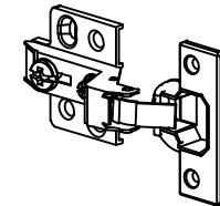
* x4 RP301603-HINGE2 Side Door Hinge Charnière de porte Bisagra de la puerta
