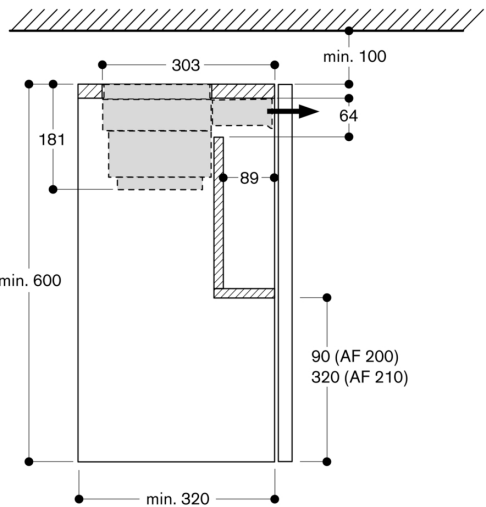
Section transversale du meuble haut avec AA 211 812
