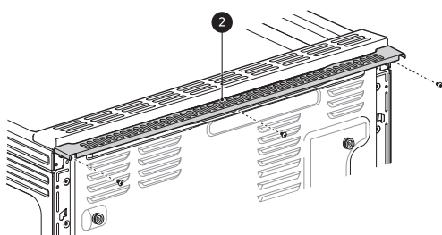
2 Placa trasera
