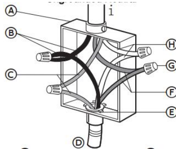
Neutro sin Conexión a Tierra
