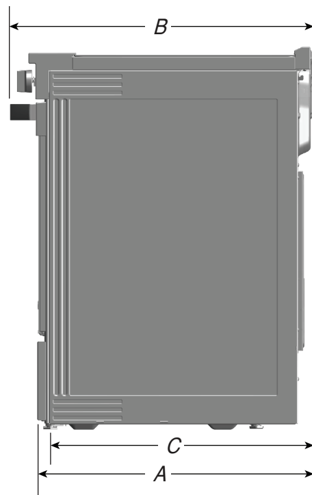
VUE LATÉRALE
