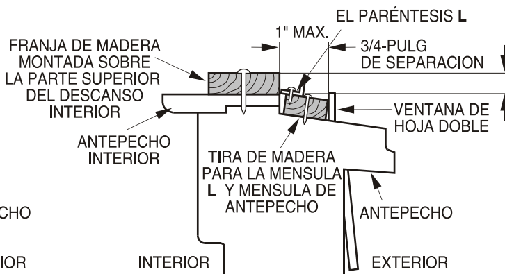
Fig. 5-2
