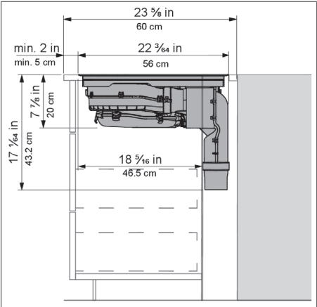
Fig. 1.2 Modelo de planificación set de recirculación
