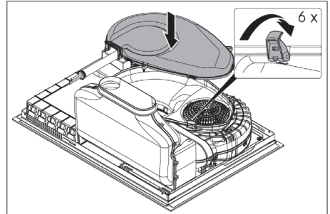
Fig. 1.7 Montaje de la carcasa de conducción del aire
