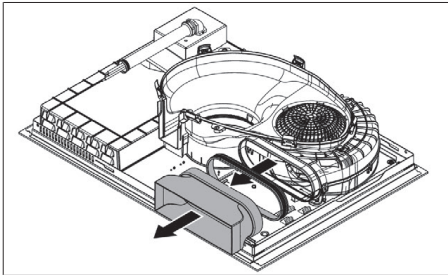
Fig. 1.5 Retrait de l'adaptateur d'air vicié
