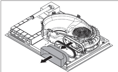
Fig. 1.5 Desmontaje del adaptador para aire de salida
