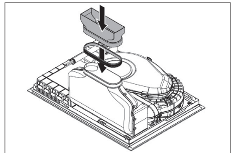
Fig. 1.8 Montage de l'adaptateur d'air vicié
