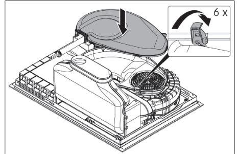
Fig. 1.7 Montage du boîtier de circulation de l'air
