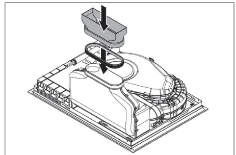
Fig. 1.8 Montaje del adaptador para aire de salida
