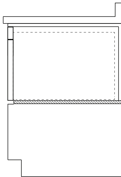
Vue latérale de l'installation encastrée
