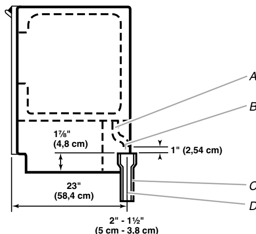
A. Tuyau de vidange B. Écart anti-retour de 1" (2,54 cm) C. Réducteur du drain de vidange PVC
