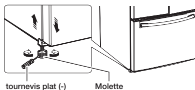
tournevis plat (-) Molette
