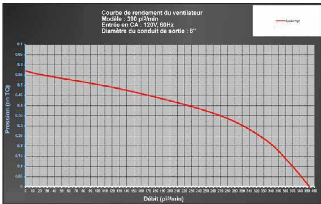
Diagrammes des courbes caractéristiques des ventilateurs
