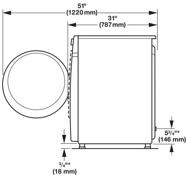
Vue latérale :
