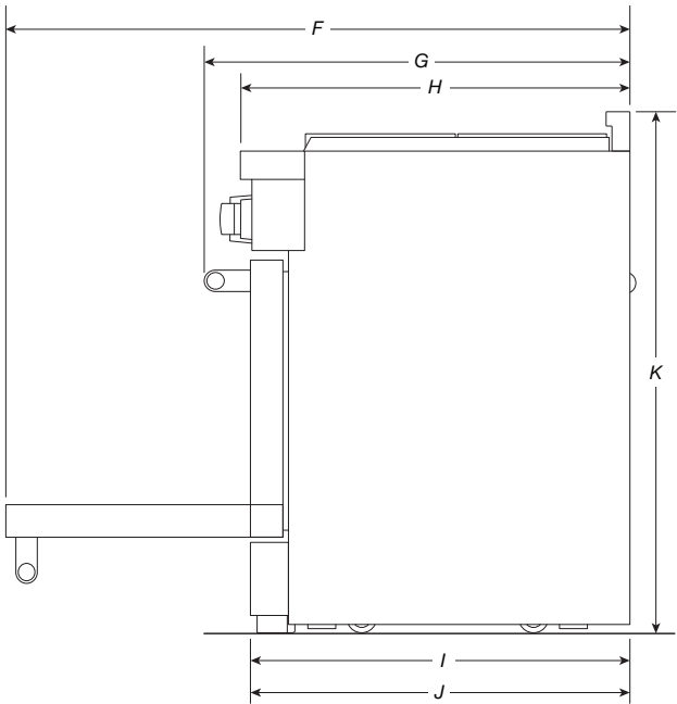
VUE LATÉRALE
