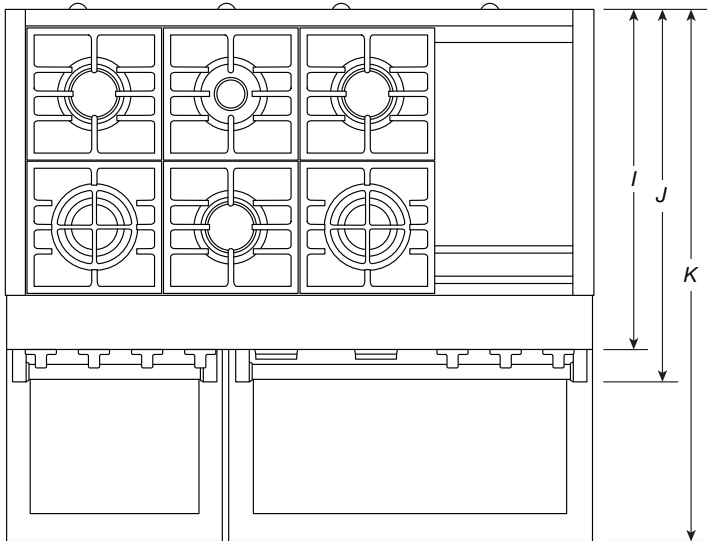
VISTA SUPERIOR
