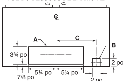
HOTTE À VENTILATEUR INTERNE SIMPLE
