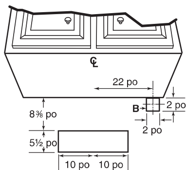
HOTTE À VENTILATEUR INTERNE DOUBLE
