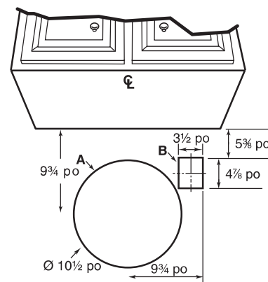
HOTTE AVEC VENTILATEUR EN LIGNE OU EXTÉRIEUR
