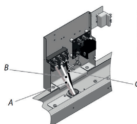
(tipo B) CONEXIÓN 3 HILOS
