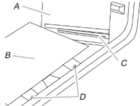
A. Miroir B. Répartiteur de flammes C. Réflexion de la flamme D. 2 vis
