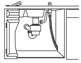
Instalación de la T de desechos
