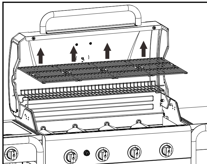
Enlever les grilles de cuisson
