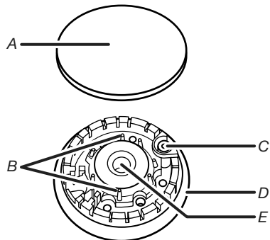
A. Chapeau de brûleur B. Tiges d'alignement C. Allumeur D. Base du brûleur E. Ouverture du tube d'arrivée de gaz
