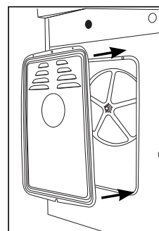
Réinstallez la plaque arrière
