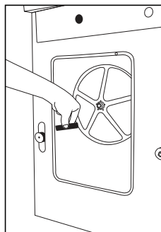
Mettez en place les entretoises de caoutchouc
