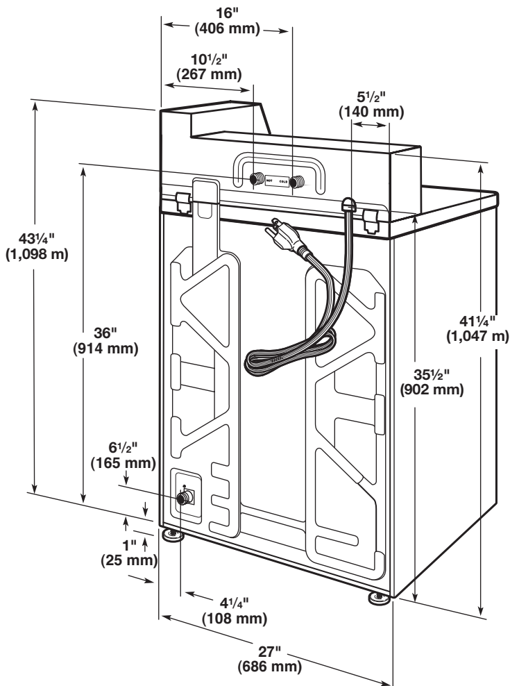
Vue arrière
