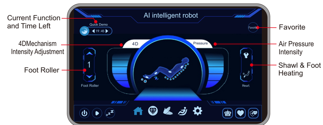
Message Interface
